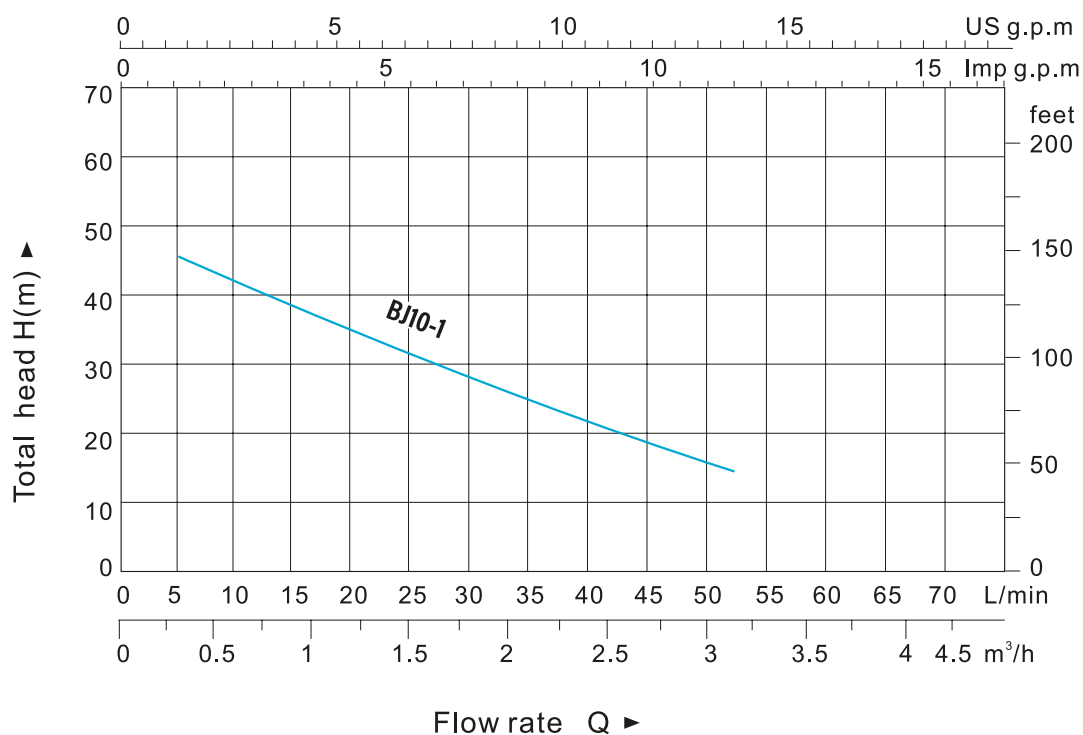
GRÁFICO DE RENDIMIENTO n=3450 rpm / 60 Hz
