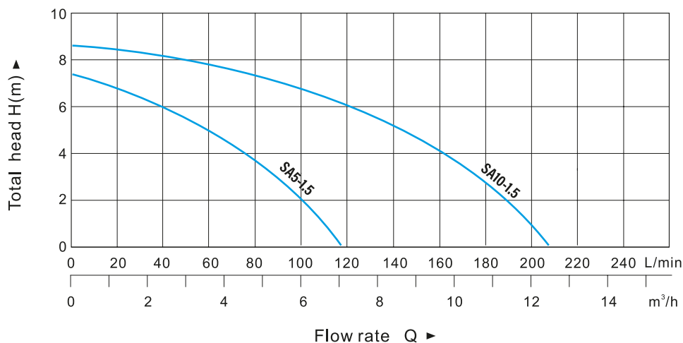
GRÁFICO DE RENDIMIENTO n=3450 rpm / 60 Hz
